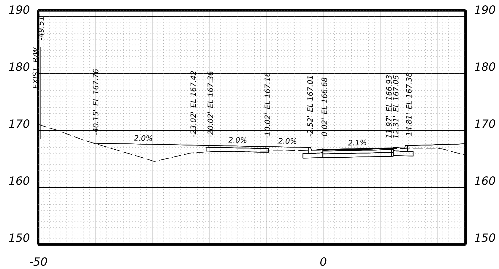
STA 33+50.00
