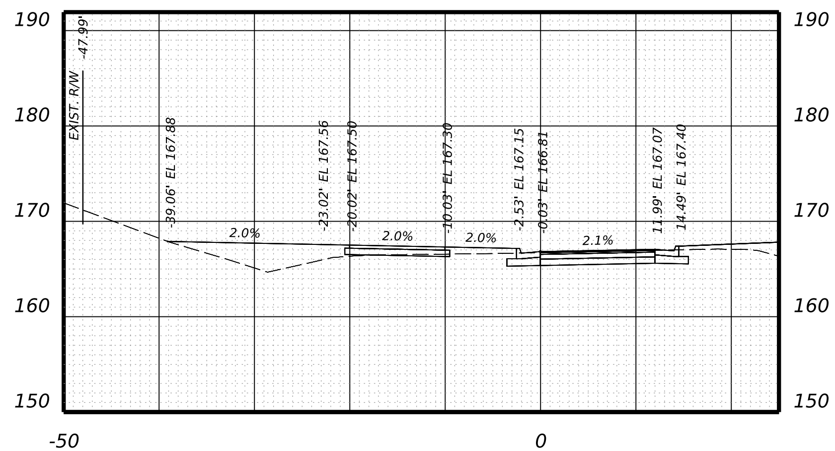
STA 33+25.00
