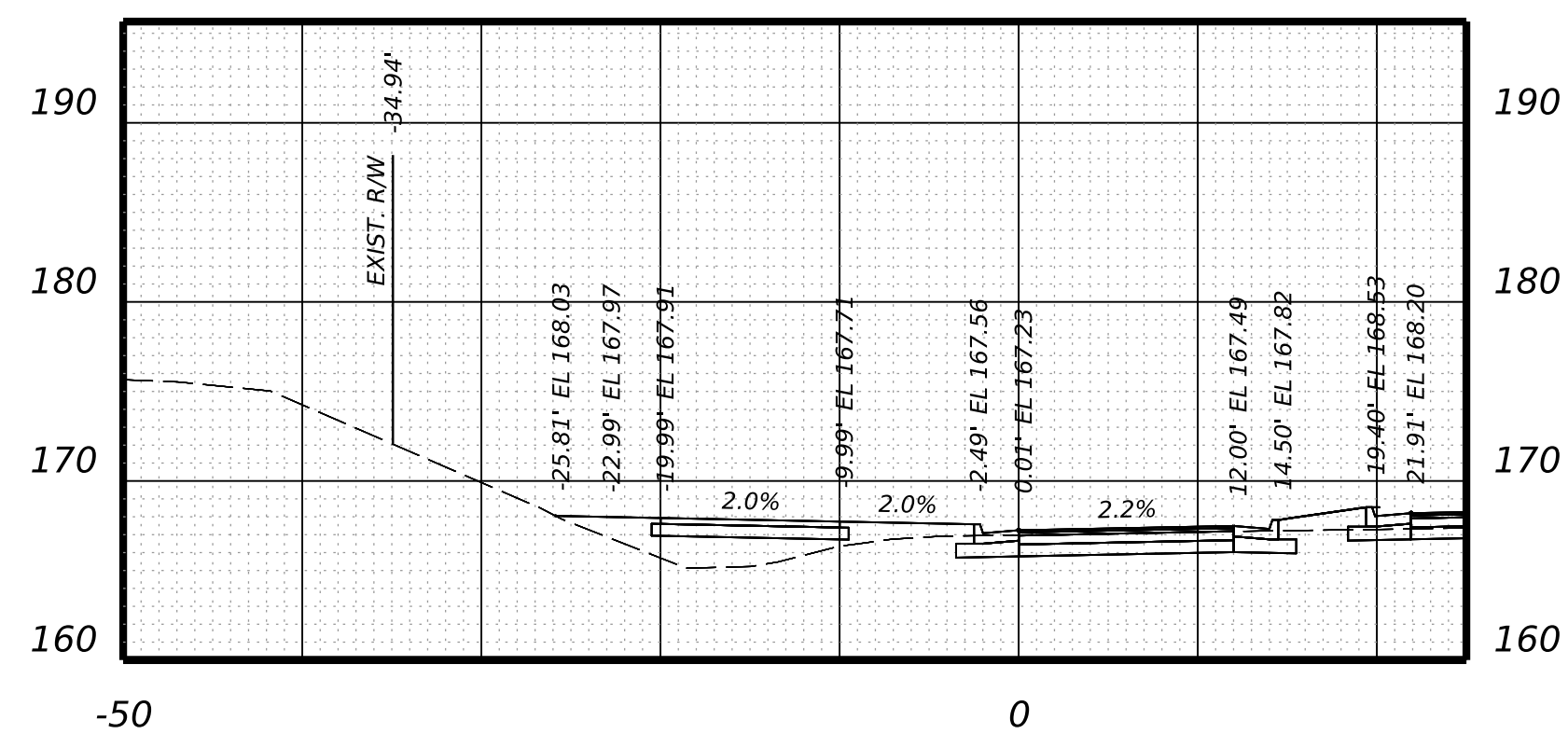
STA 32+50.00
