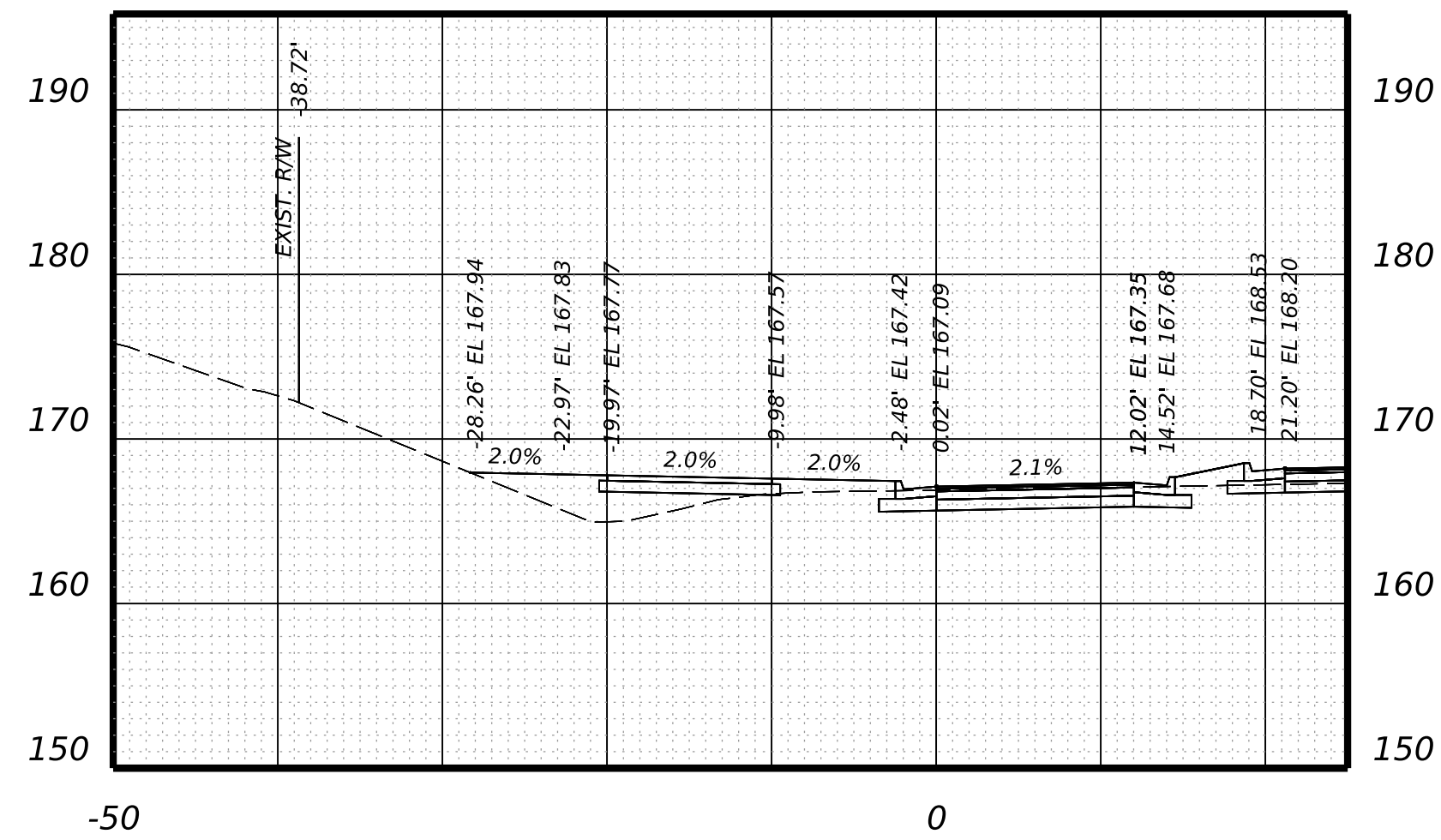
STA 32+75.00
